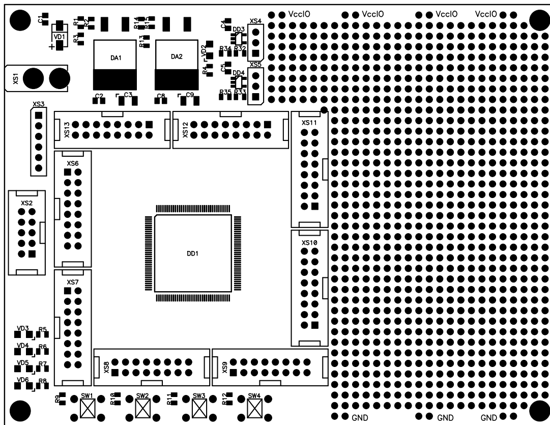
Рис. 4. Внешний вид печатной платы
