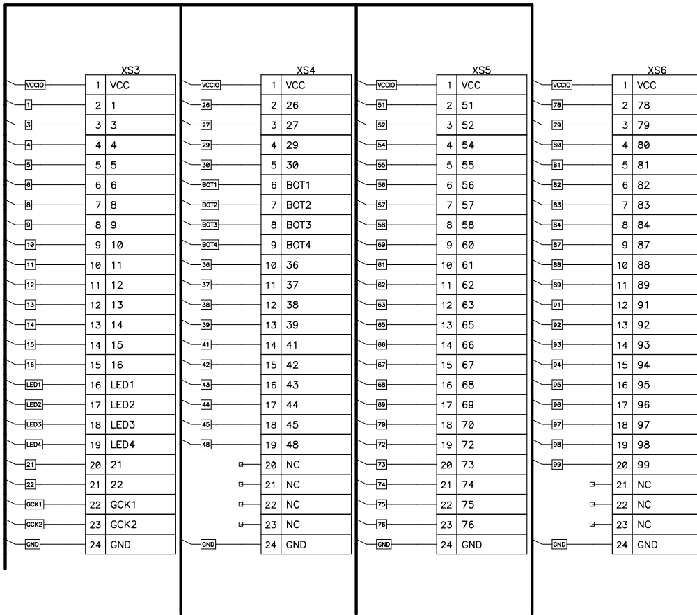
Рис. 2. Схема электрическая принципиальная XB-XC9572-PQ100 (Продолжение)
