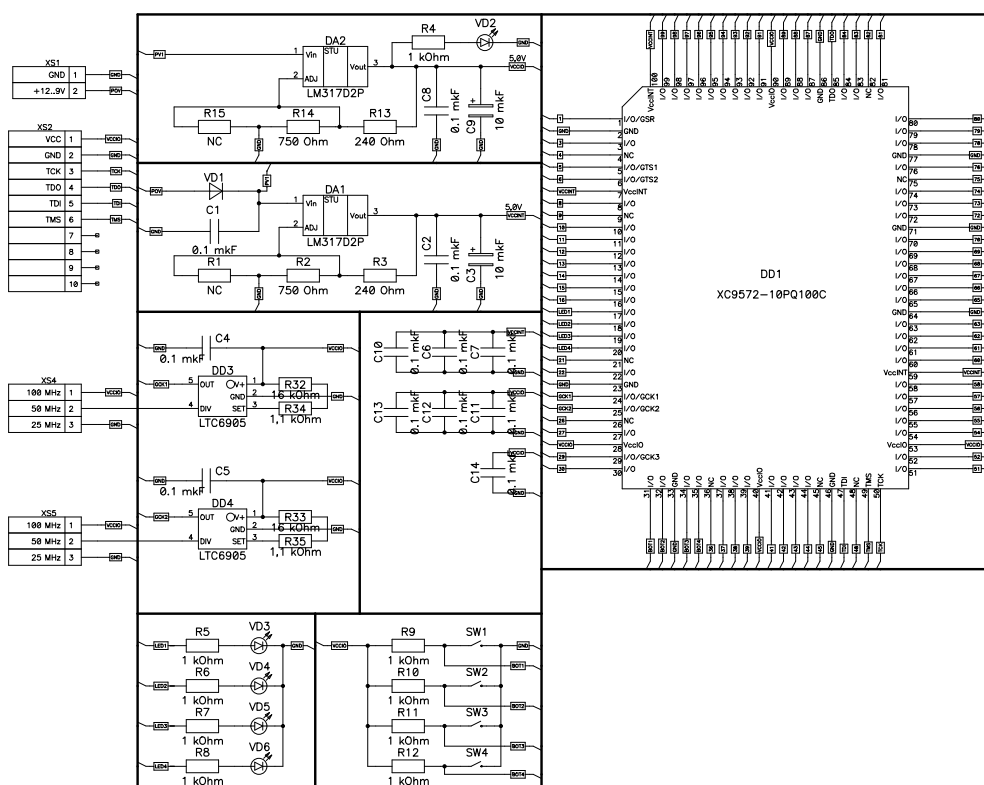
Рис. 2. Схема электрическая принципиальная XB-XC9572-PQ100
