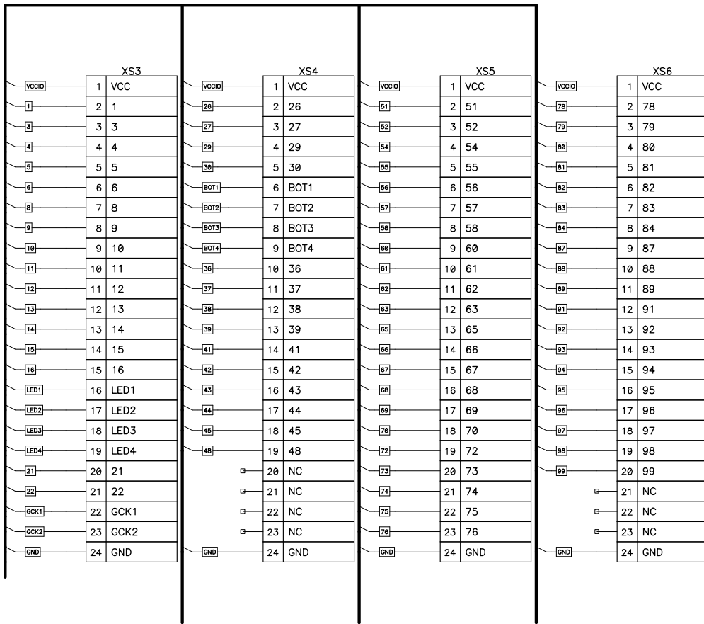
Рис. 3. Схема электрическая принципиальная XB-XC95108-PQ100
