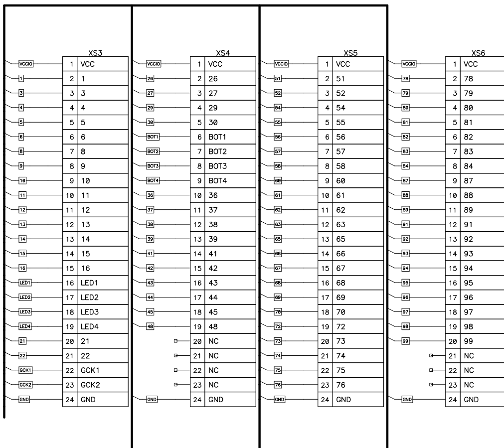
Рис. 4. Схема электрическая принципиальная XB-XC95144-PQ100 (Продолжение)
