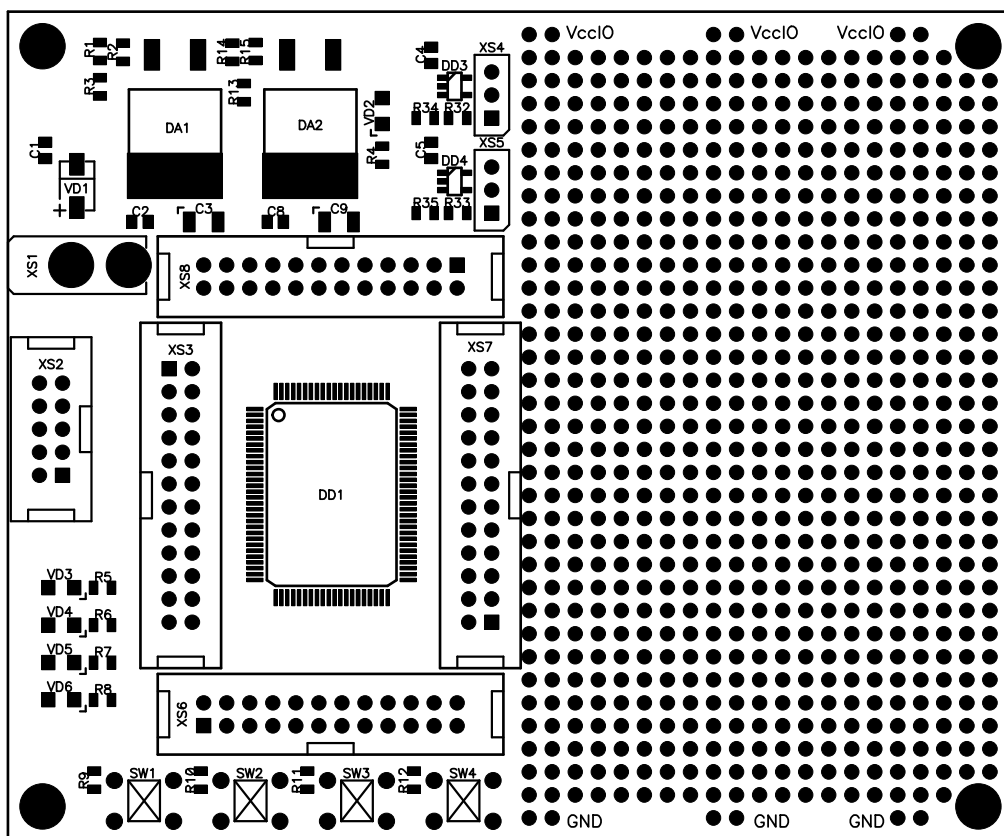
Рис. 5. Внешний вид печатной платы
