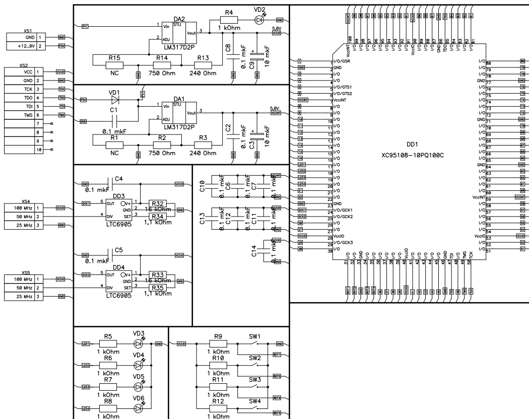
Рис. 3. Схема электрическая принципиальная XB-XC95108-PQ100
