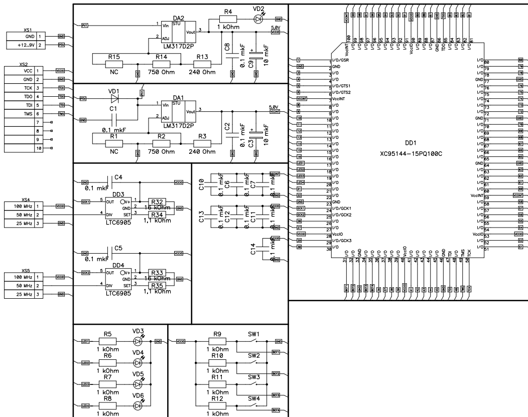
Рис. 4. Схема электрическая принципиальная XB-XC95144-PQ100
