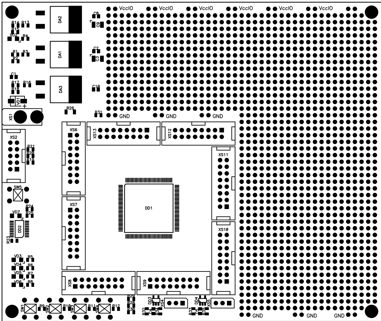
Рис. 6. Внешний вид печатной платы конструктора-ПЛИС
